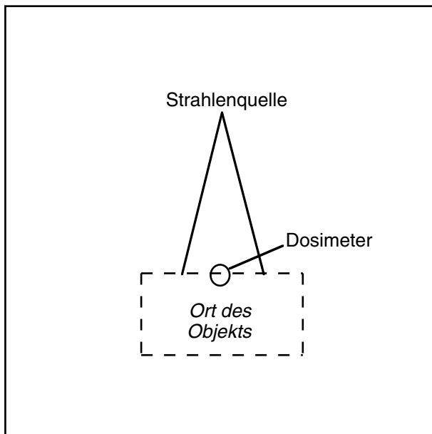
Abb. 7.2 Einfalldosis.
