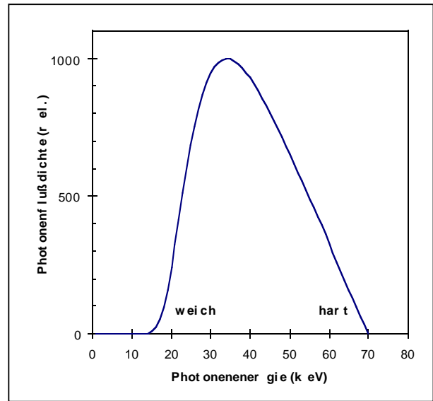
Abb. 2.3 Typisches Strahlenspektrum in der Röntgendiagnostik (Wolfram-Anode, 70 kV Röhrenspannung, Filterung mit 2,5 mm Aluminium).
