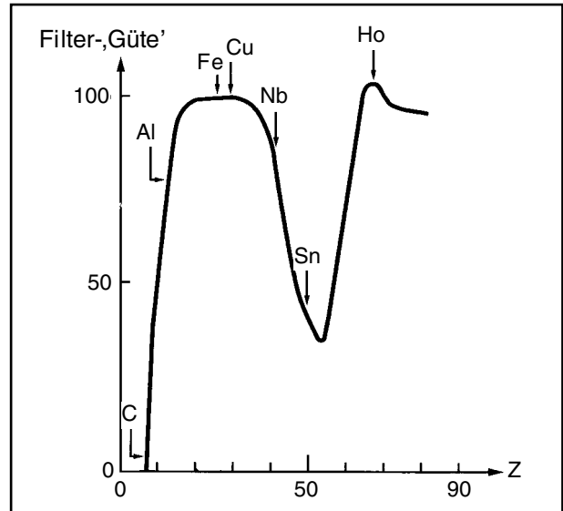
Abb. 4.6 Filter-,Güte' unterschiedlicher Materialien als Funktion ihrer Ordnungszahl Z bei 70 kV Röhrenspannung.
