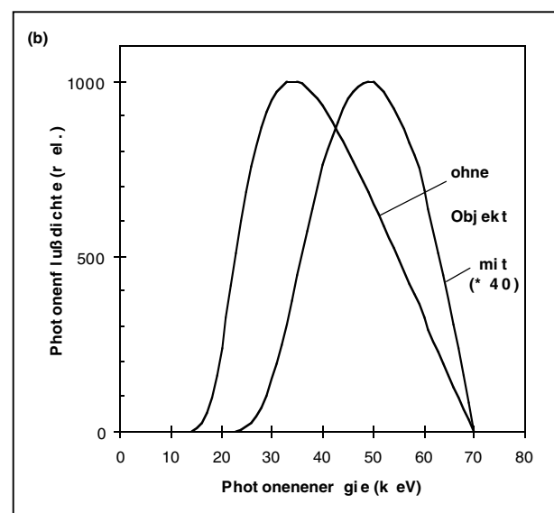
Abb. 5.1 Röntgenspektrum - Schwächung (a) und Aufhärtung (b) im Objekt (15 cm Gewebe).
