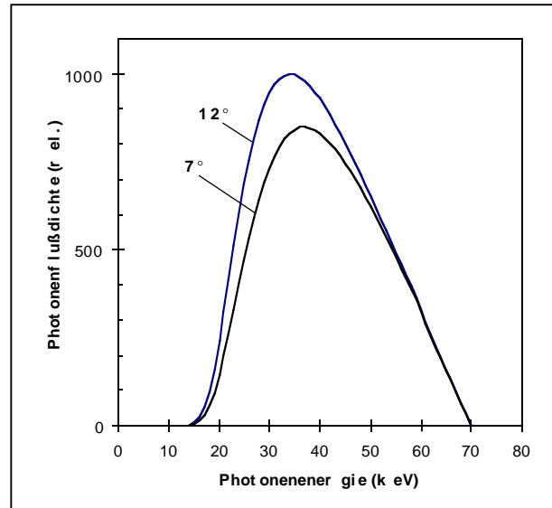
Abb. 2.11 Röntgenspektrum - Einflußgröße Anodenwinkel ( 12^\circ , 7^\circ ).
