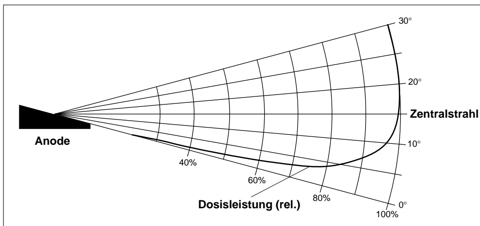
Abb. 2.10 Heeleffekt bei einer Röntgenröhre mit 15^\circ Anodenwinkel.
