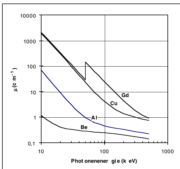
Abb. 4.4 Schwächungscharakteristik (linearer Schwächungskoeffizient \mu ) unterschiedlicher Filtermaterialien.
