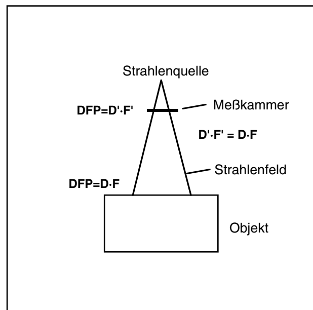
Abb. 7.5 Dosisflächenprodukt (DFP).
