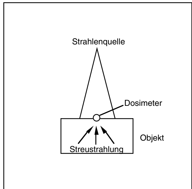
Abb. 7.3 Oberflächendosis.
