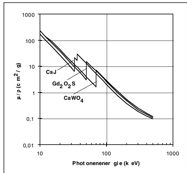
Abb. 6.5 Absorptionscharakteristik (Massenschwächungskoeffizient \mu/p ) einiger Bildempfängermaterialien.
